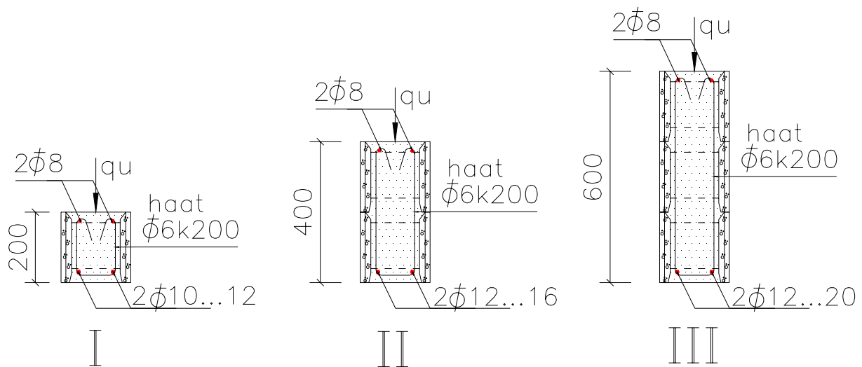
Kuva 11. Leikkausraudoitettu palkki
