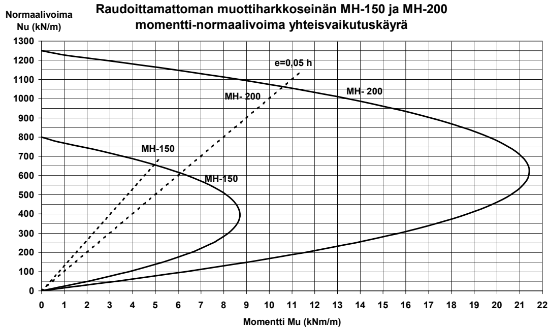
Kuva 7. Harkkoseinän pystykuorman ja taivutusmomentin yhteisvaikutuskäyrä Laskentakuorman aiheuttama momentti-normaalivoima-yhdistelmä ( M_d , N_d ) tulee sijaita käyrän sisäpuolella (käyrän ja pysty akselin rajaamalla alueella).
