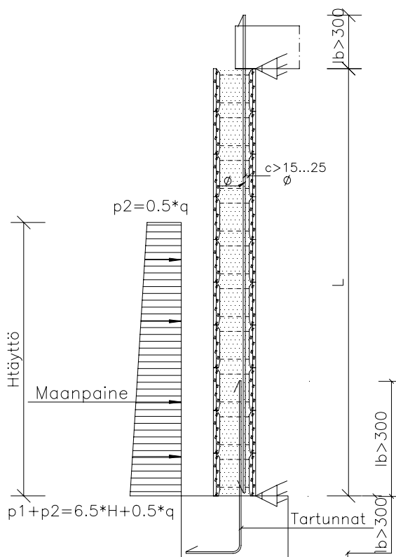
Kuva 8. Pystyterästen sijoitus maanpaineseinässä.
