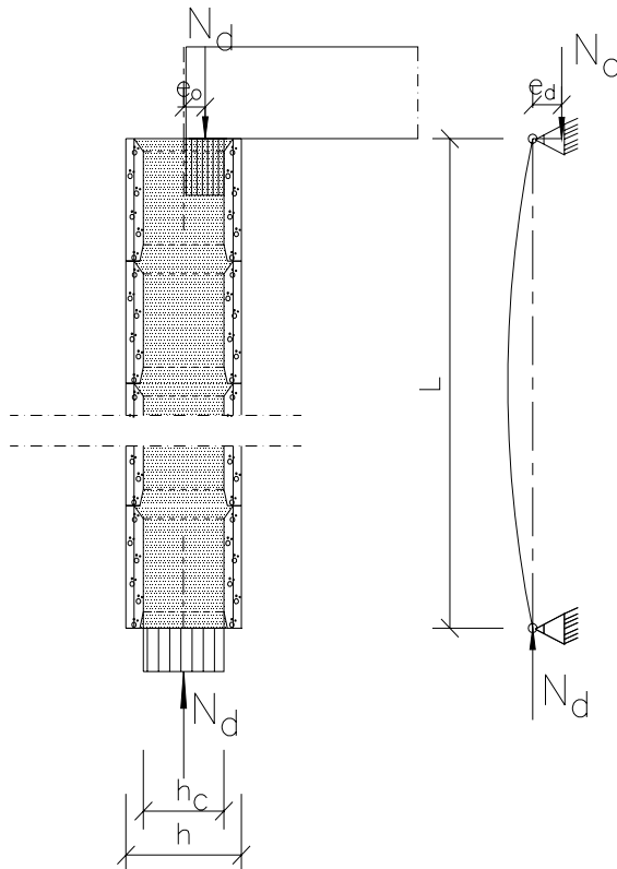
Kuva 5. Seinän staattinen malli ja pystykuorman epäkeskisyyys.
