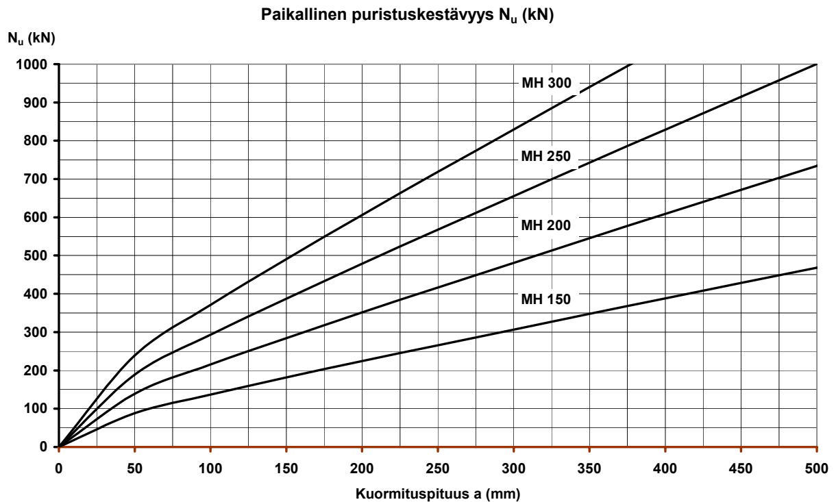
Kuva 12. Paikallinen puristuskestävyys
