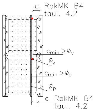
Kuva 4. Betonipeite
